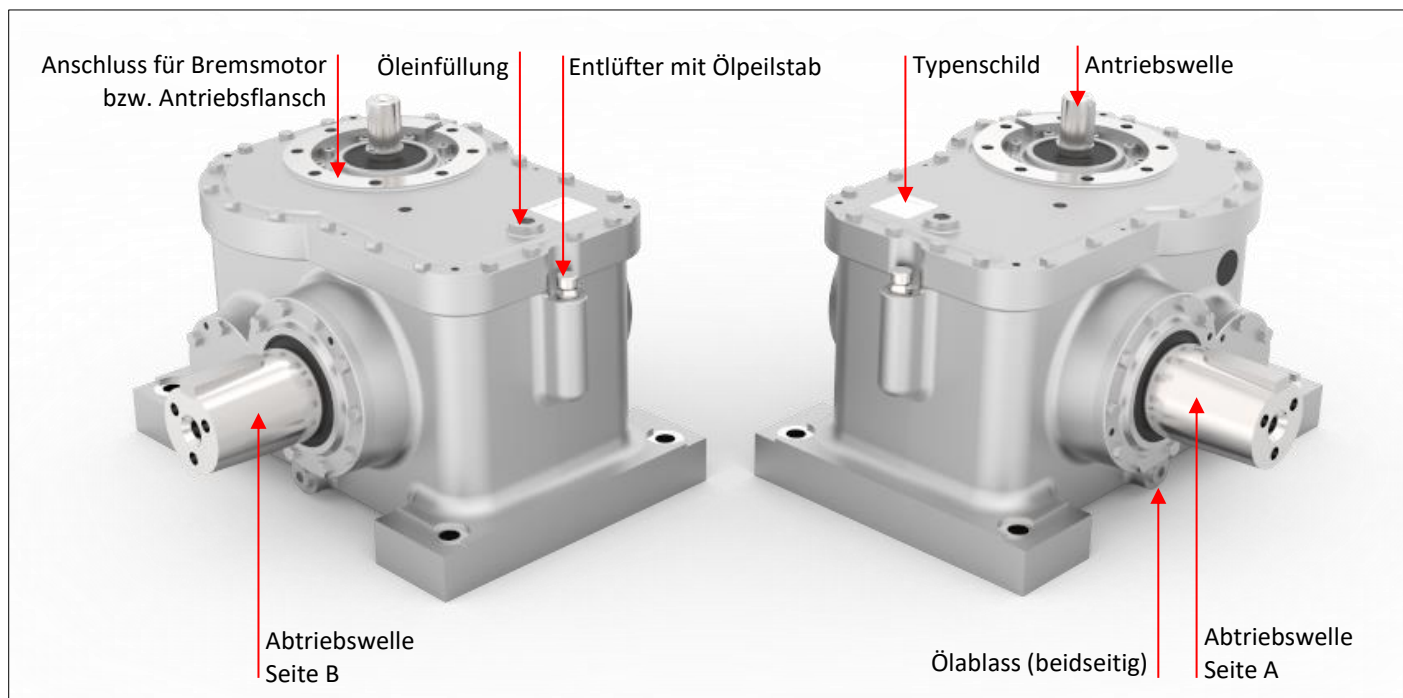
Abbildung 3.1-1: Aufbau Basisversion am Beispiel FTHST168.1
