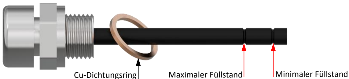
Abbildung 3.3.3: Entlüfter mit Ölpeilstab
