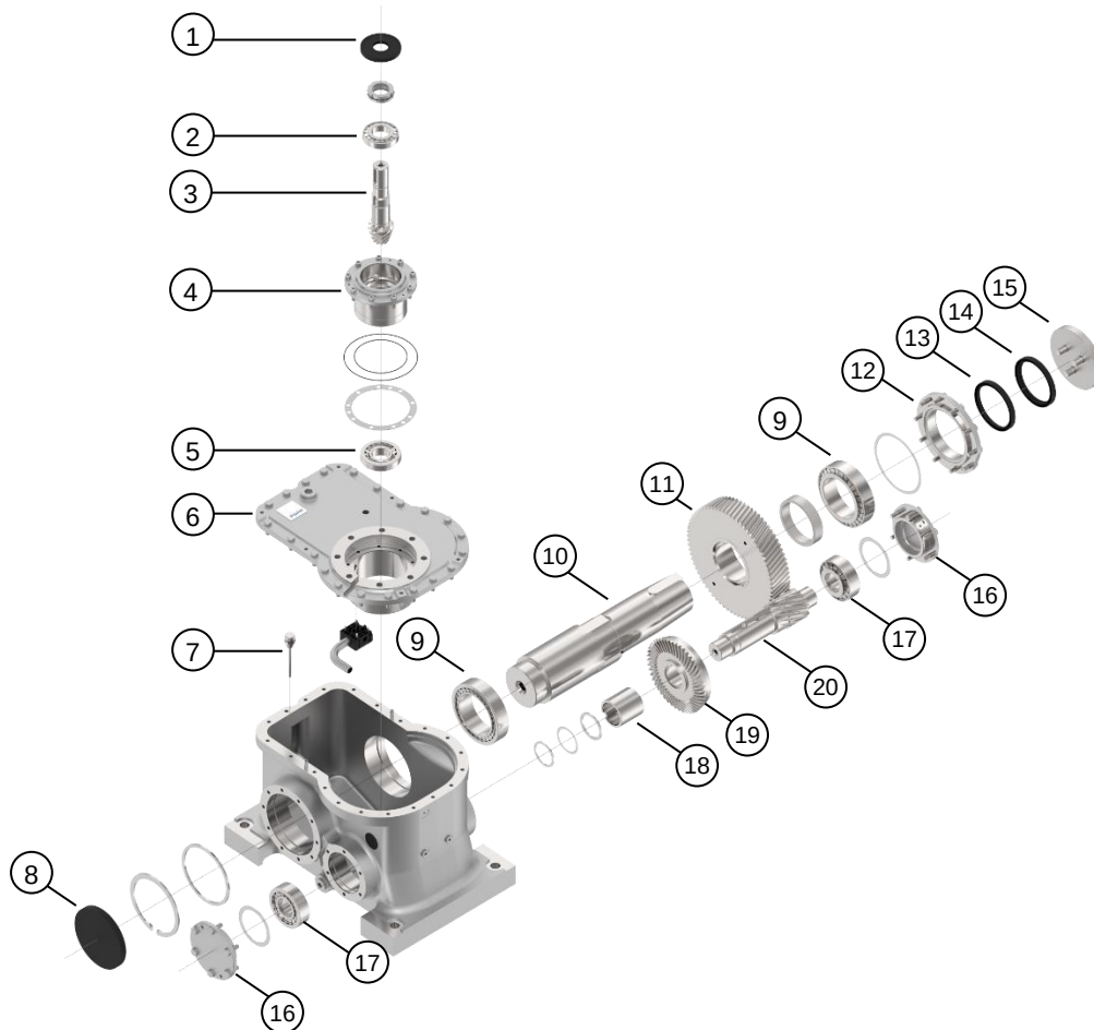
Abbildung 8.2: Explosionsdarstellung (Beispiel FTHST168.1)
