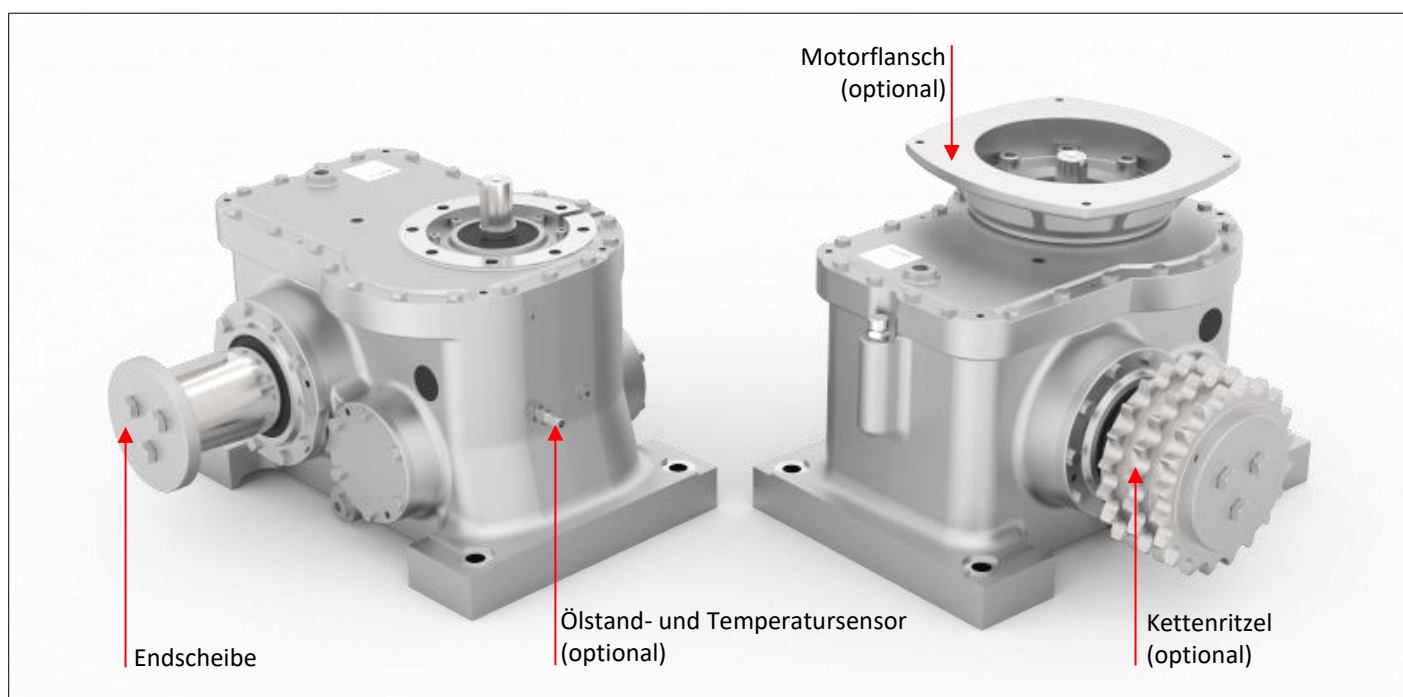
Abbildung 3.1-2: Anbau-Optionen am Beispiel FTHST168.1
